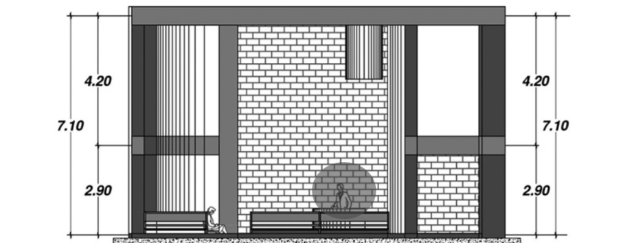
CORTE Y - Y' Capilla Ibero
